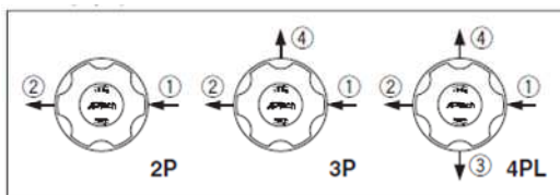
①IN ②OUT ③④OUT側ゲージポート
