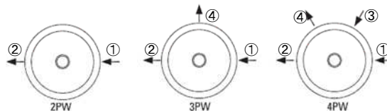
①IN ②OUT ③IN側ゲージポート ④OUT側ゲージポート
